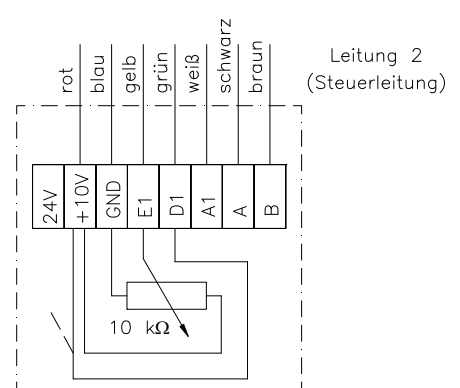
Drehzahlsteller
