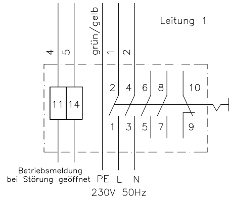
Reparaturschalter
