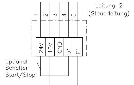
Klemmkasten
