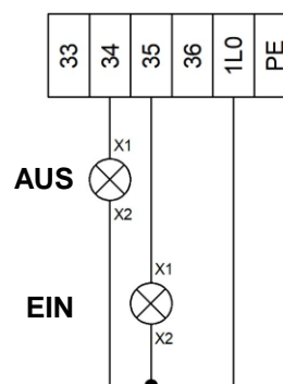
Betriebsmeldung Absaugung 3
